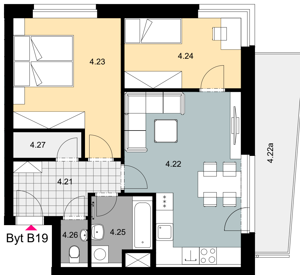
Schéma bytu
