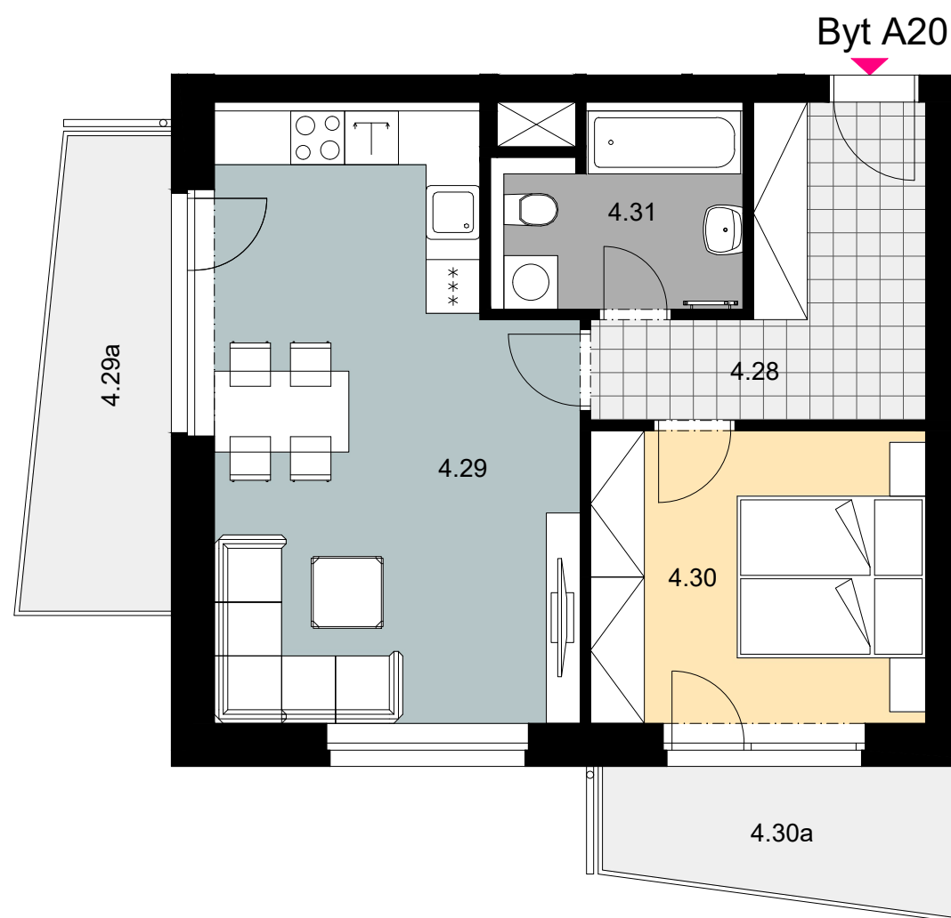
Schéma bytu
